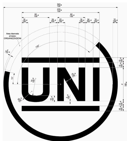
GRIGLIA DI COSTRUZIONE DEL MARCHIO UNI
